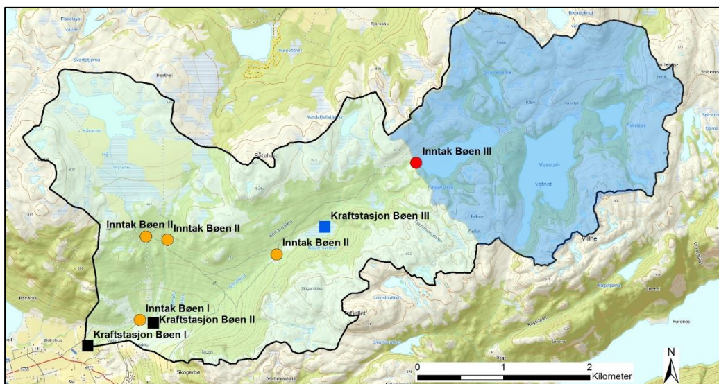
Figur 5.1. Nedbørfelt til den nederste kraftstasjonen (Bøen I) og til planlagt reguleringsdam ved Kaldavatnet (mørkere blå).
