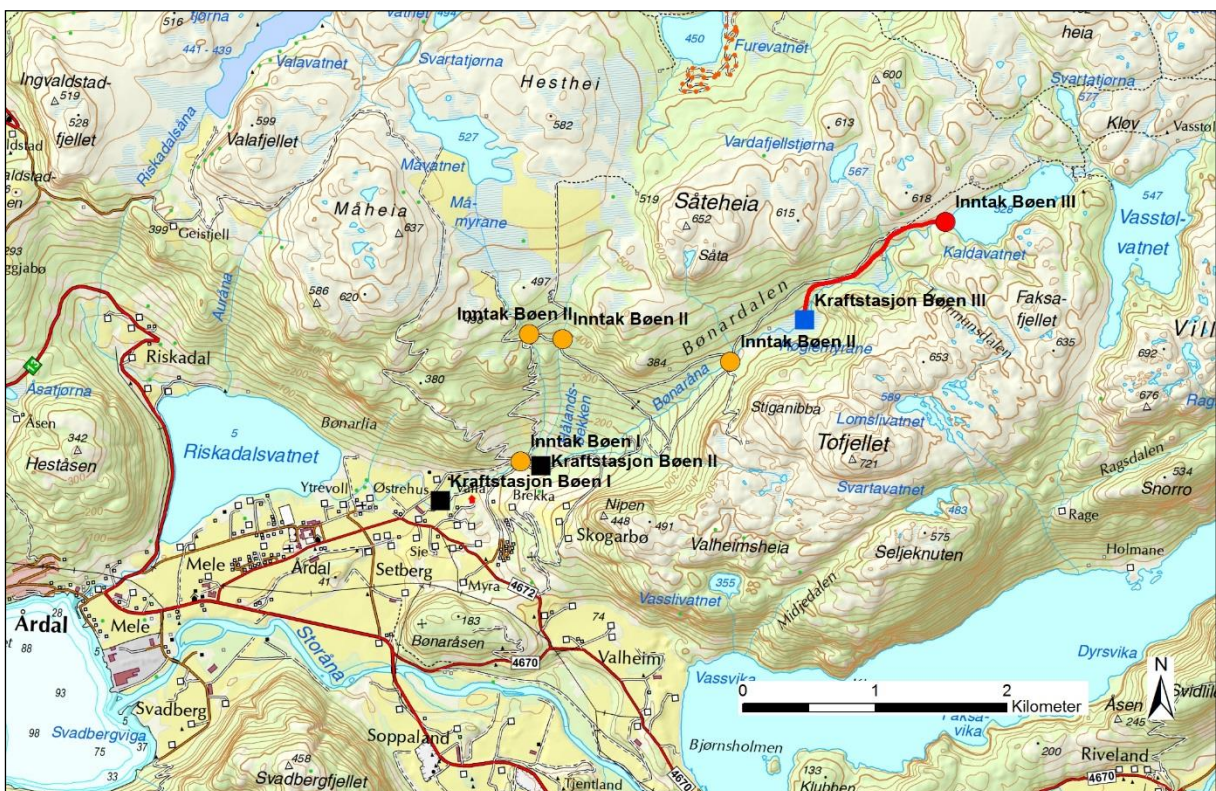
Figur 2.2. Oversikt over planlagte og eksisterende vannkraftprosjekt i Bøen. Lokalisering av planlagt dam (rød prikk) og ny kraftstasjon (blå firkant). Rød linje er trasé for rørgate. Eksisterende inntak og kraftstasjoner er vist med oransje prikker og svarte firkanter.
