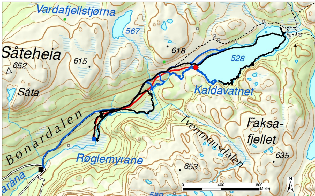
Figur 3.4. Befaringsrute (blå linje: 8. november 2018, svart linje: 27. juni 2019). De planlagte tiltakene er vist med rødt punkt for inntak/dam, blå firkant for kraftstasjon og rød linje for rørgate. Svart firkant viser inntak for kraftverket Bøen II.
